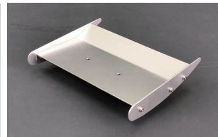
AC0501# ビンテージバギージュラウイング税別予価 ¥3500 ※ウイング固定穴ピッチは 30 ミリなので、ターボスコピオン等ではシャシー側のウイングマウントにダイレクトに取付けできません。
